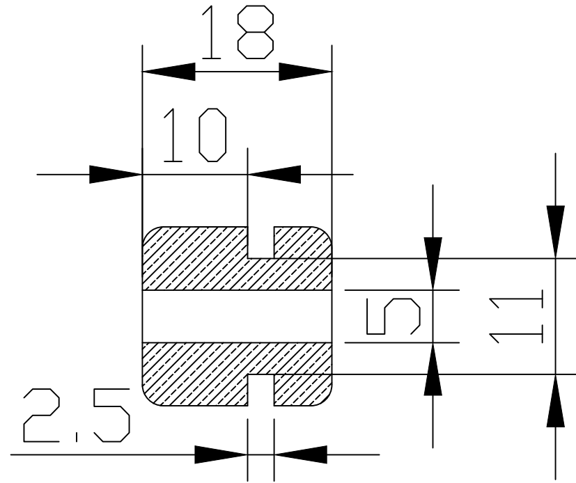
Sezione A-A
